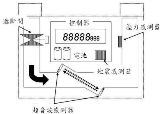
圖 B.1 超音波氣量計構造之參考圖例
