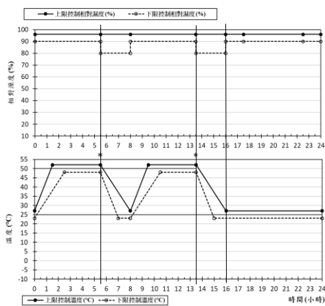
*：表示在此點容許的誤差為±5分鐘 圖 B.4.2 不含低溫之 24 小時循環
