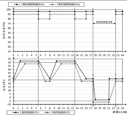
*：表示在此點容許的誤差為±5分鐘 圖 B.4.1 含低溫之 24 小時循環
